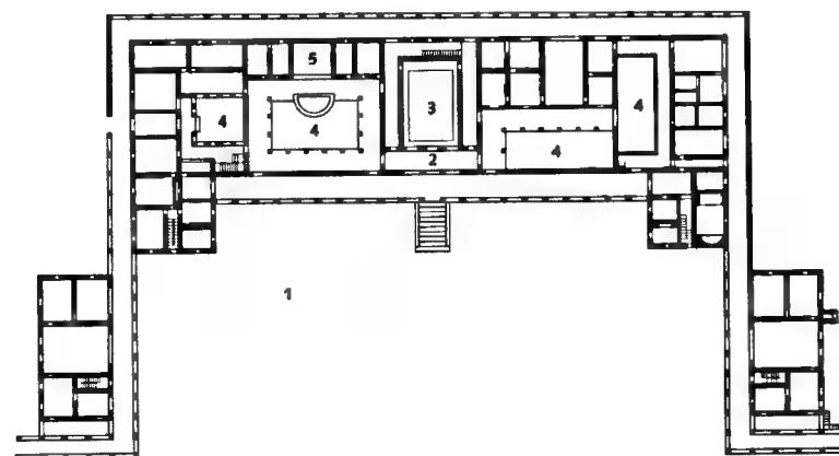
Boscoreale, Villa della Pisanelia; 1. Jh. v. Chr. (Grundriß).
